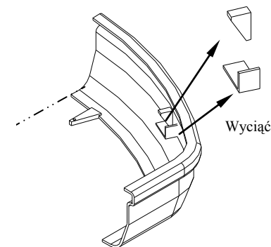
Rys. 2 Wycięcia zderzaka
